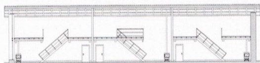
Sección A-A'
